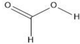
Abb. 1: Ameisensäure
